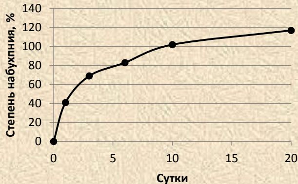
Рис. 1 – Изменение степени набухания резины:
